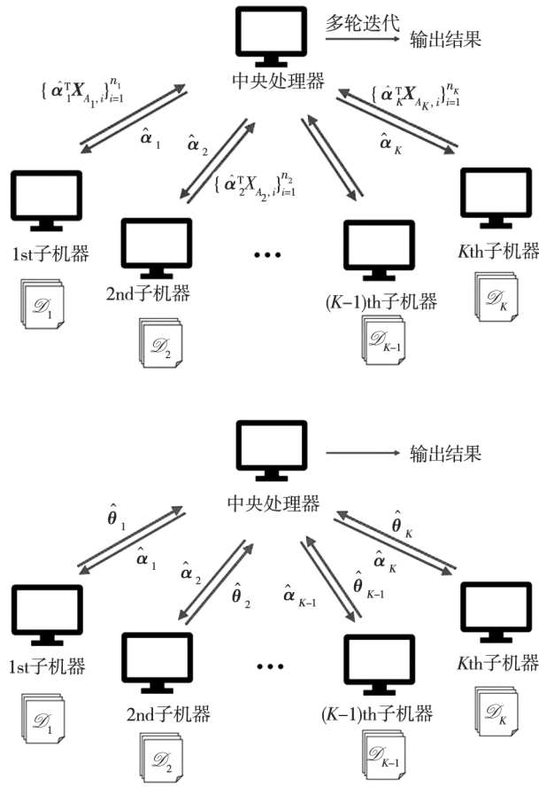
图 3 非平衡半监督数据的通讯有效算法示意图
