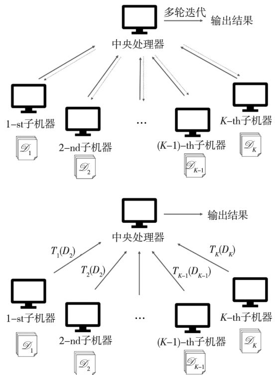
图 1 分块集成算法(上)与数萃算法(下)的算法示意图
